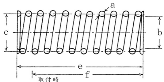
押しバネ参考図
